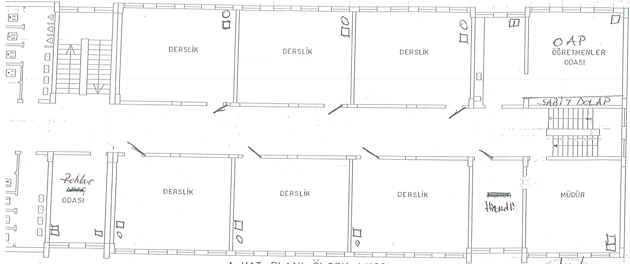
1. KAT PLANI ÖLÇEK: 1/100
